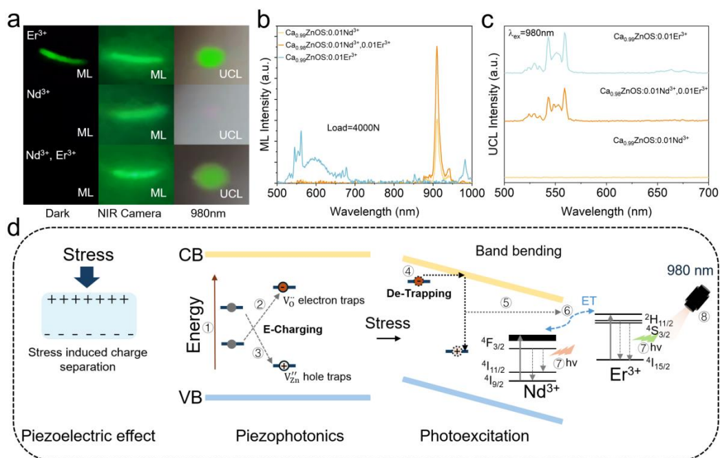
图 2 基于 \text{CaZnOS: Nd}^{3+}, \text{Er}^{3+} 材料的发光性能及应力发光机理
