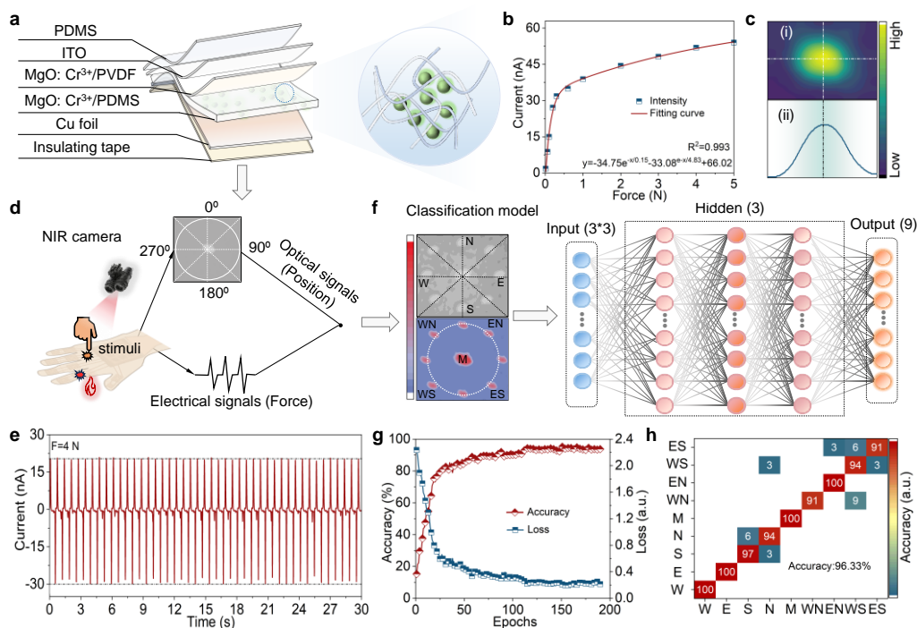
图3 (a) 多层结构传感器: MgO: Cr 3+ /PDMS 和 MgO: Cr 3+ /PVDF 被包裹在铜膜和 ITO 膜 (b) MgO: Cr 3+ 的稳定电流输出从 0.01 到 5N (c) 光学信号输出的传感器 (d) 多层柔性结构中的原位光电输出原理图以及相应概念验证触觉传感系统的应用 (e) 在持续机械刺激下传感器的电学循环测试 (f) 九个不同位置的 ML 图片以及相应的二维空间光学映射和神经网络架构 (g) 识别准确率和损失函数。(h) 九个不同位置的预测的混淆矩阵
