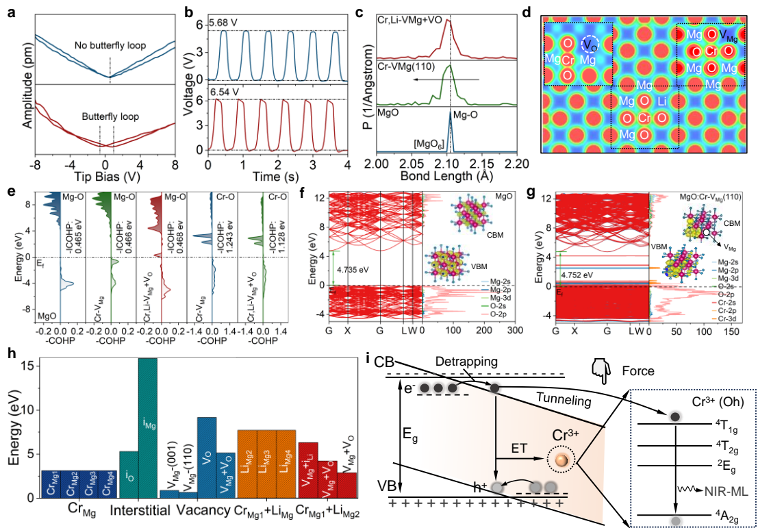
图 2 (a) \text{Mg}_{0.999}\text{O}:0.001\text{Cr}^{3+} 和 \text{MgO} 的 PFM 的振幅和蝴蝶曲线 (b) \text{Mg}_{0.999}\text{O}:0.001\text{Cr}^{3+} 和 \text{MgO} 的稳定电压输出 (c) 不同的计算模型下的 \text{Mg-O} 键长分布 (d) 电荷分布的二维切片 (e) 不同模型下的 COHP 曲线 (f) \text{MgO} 的能带、电子态密度和费米能级 (g) \text{MgO}:\text{Cr} 的能带、电子态密度和费米能级 (h) 不同类型缺陷的形成能 (i) ML 机理示意图
