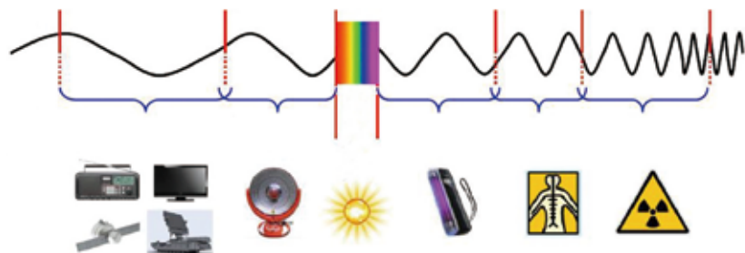
图 5-1 电磁波谱与辐射类型的关系
