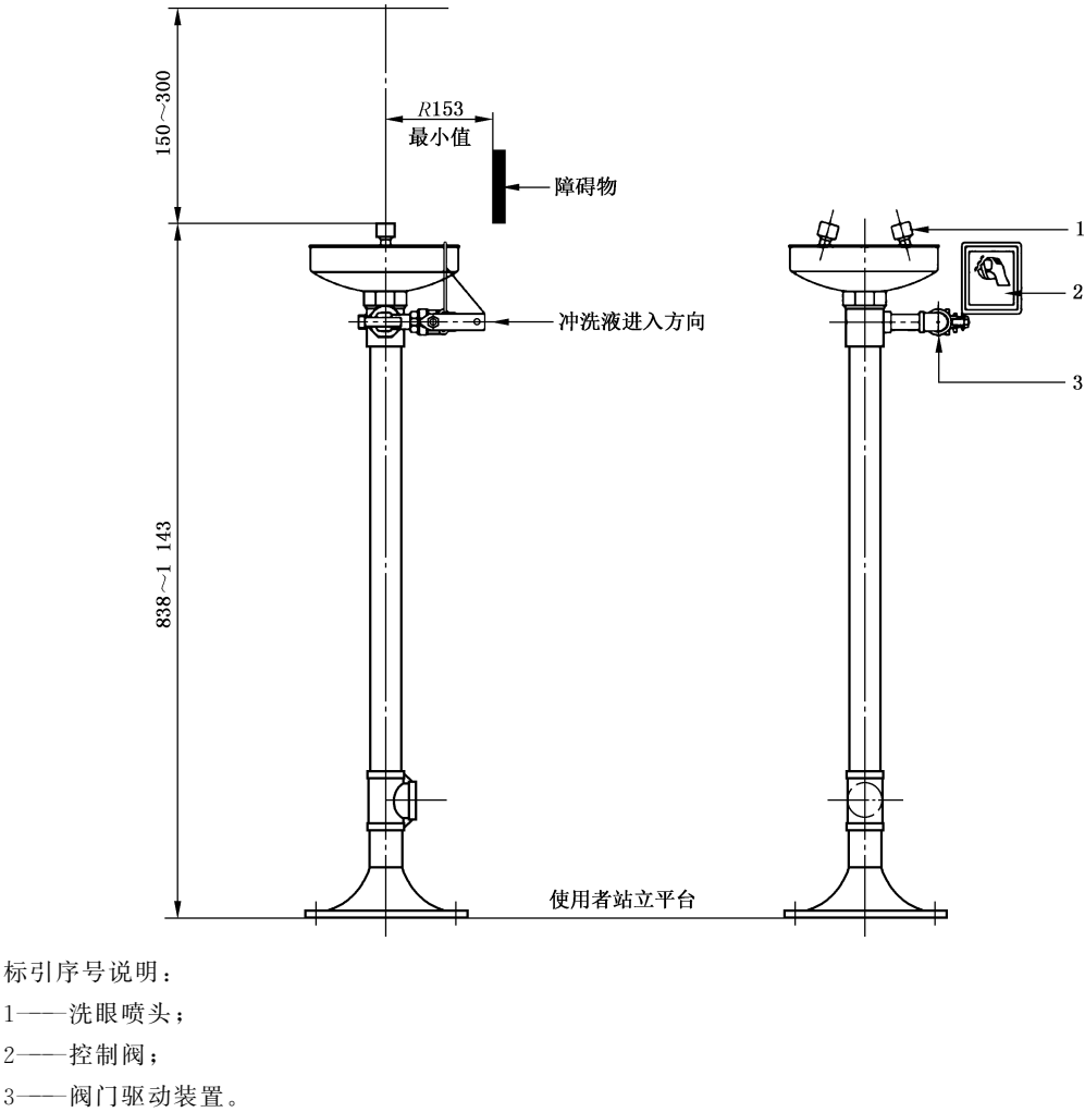
图 3 洗眼器示意图
