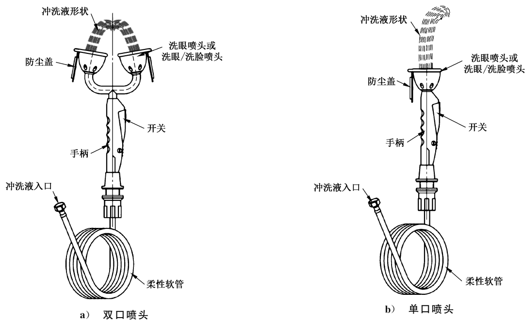
图 A.1 喷淋软管示意图
