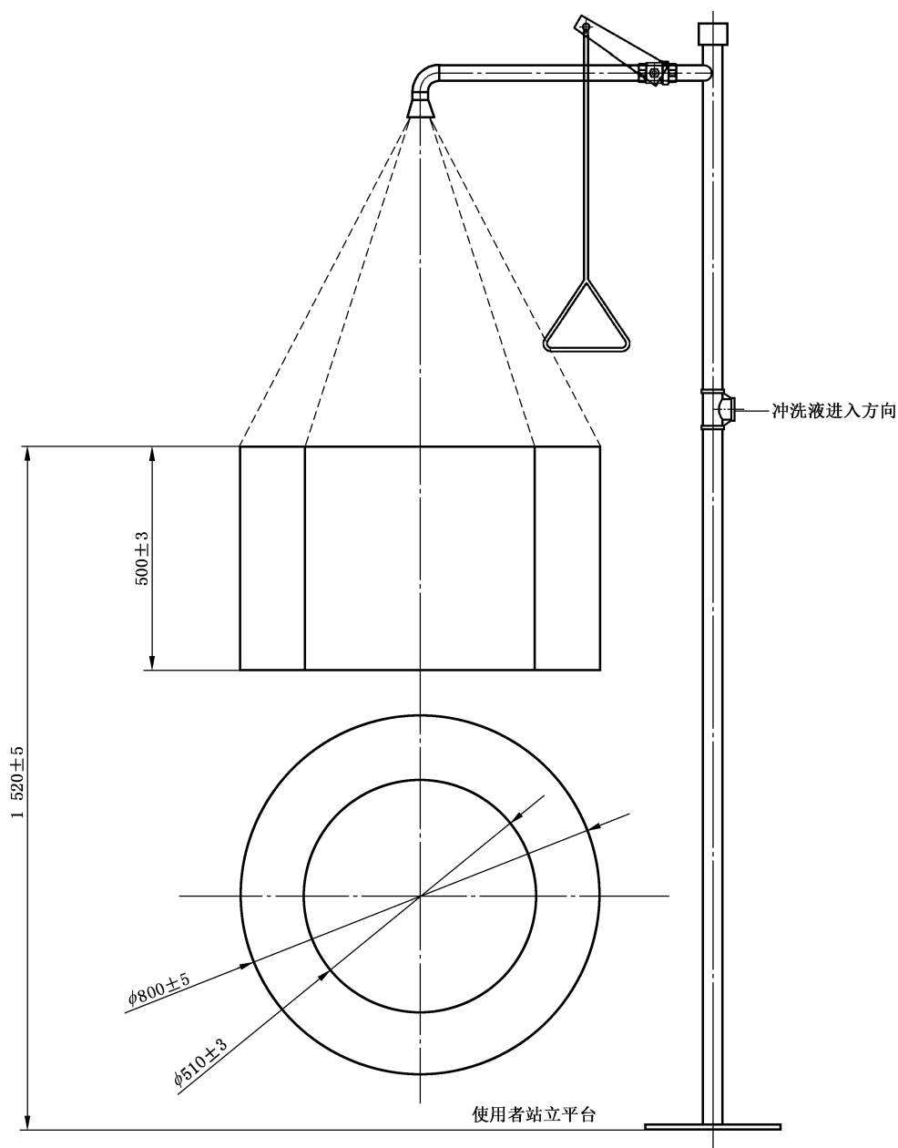
图2 冲洗液分散性测试示意图
