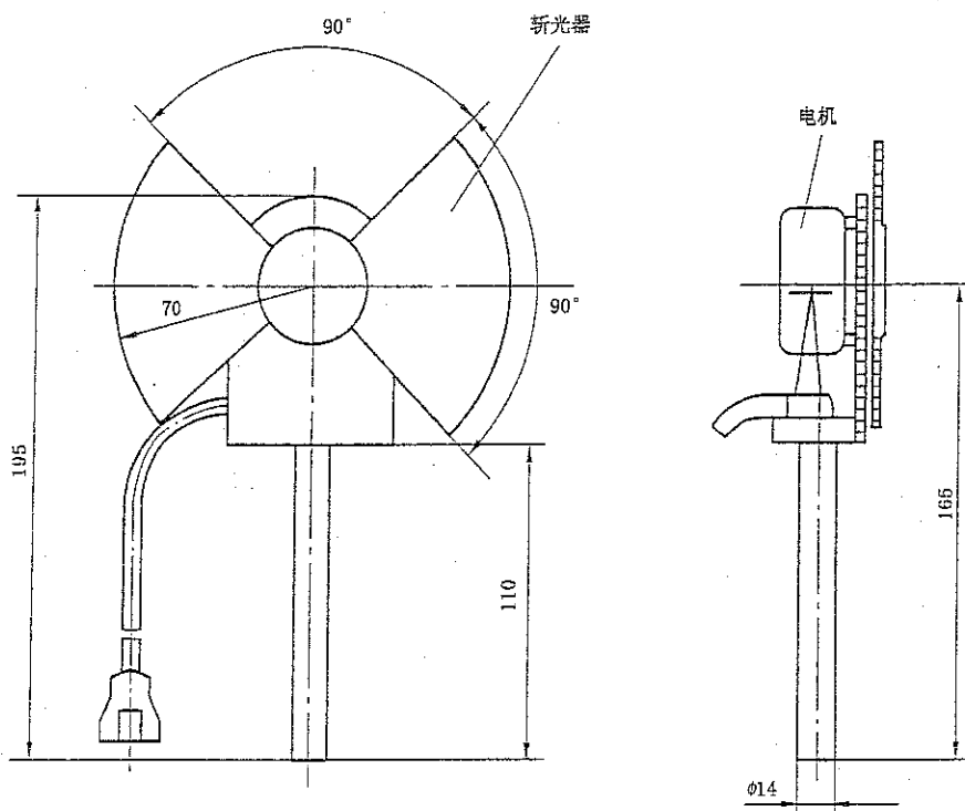
图2 调制器结构图
