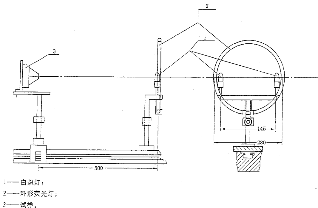
图 5 环境光干扰试验装置结构图
