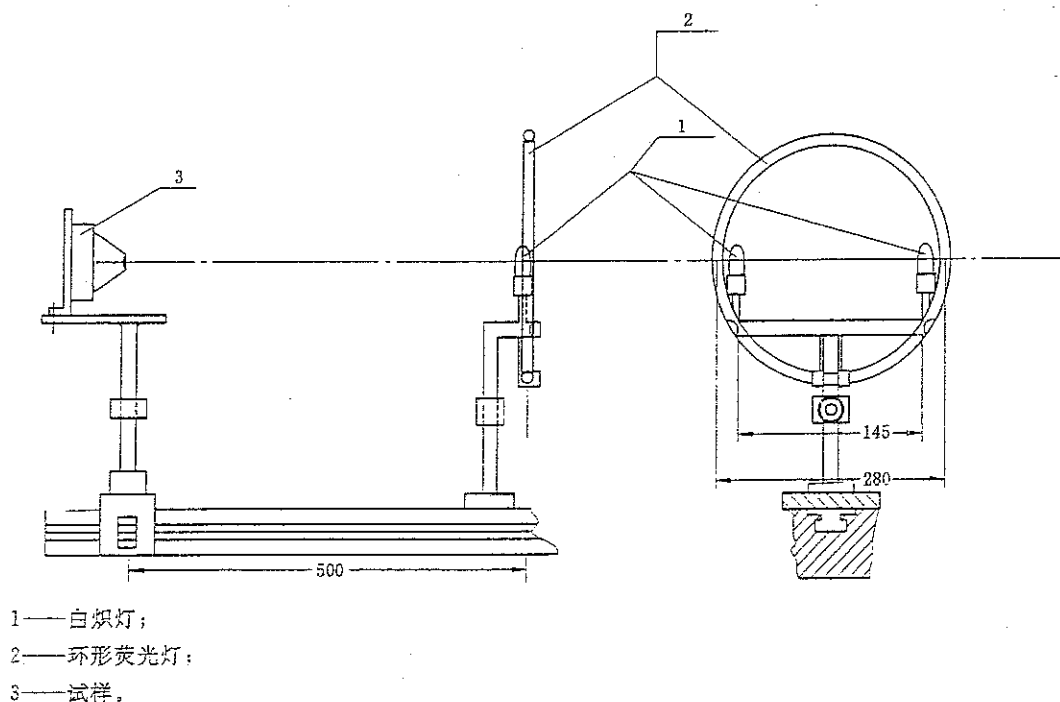
图 3 环境光线干扰模拟装置结构图
