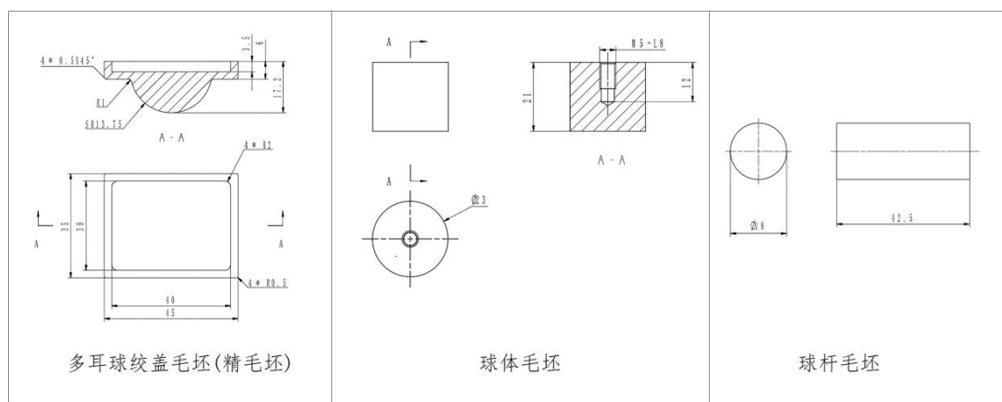
图 9 毛坯尺寸图 (精毛坯表面粗糙度 Ra3.2)
