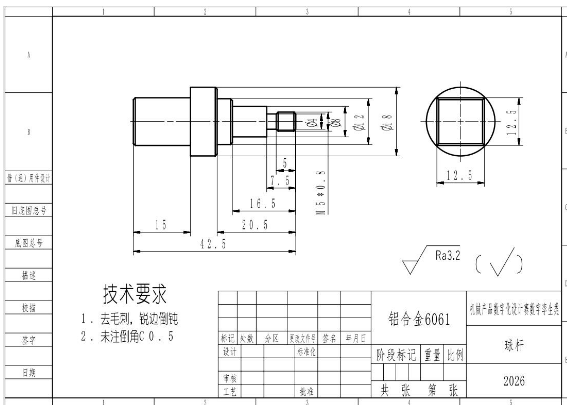
图 8 球杆工程图
